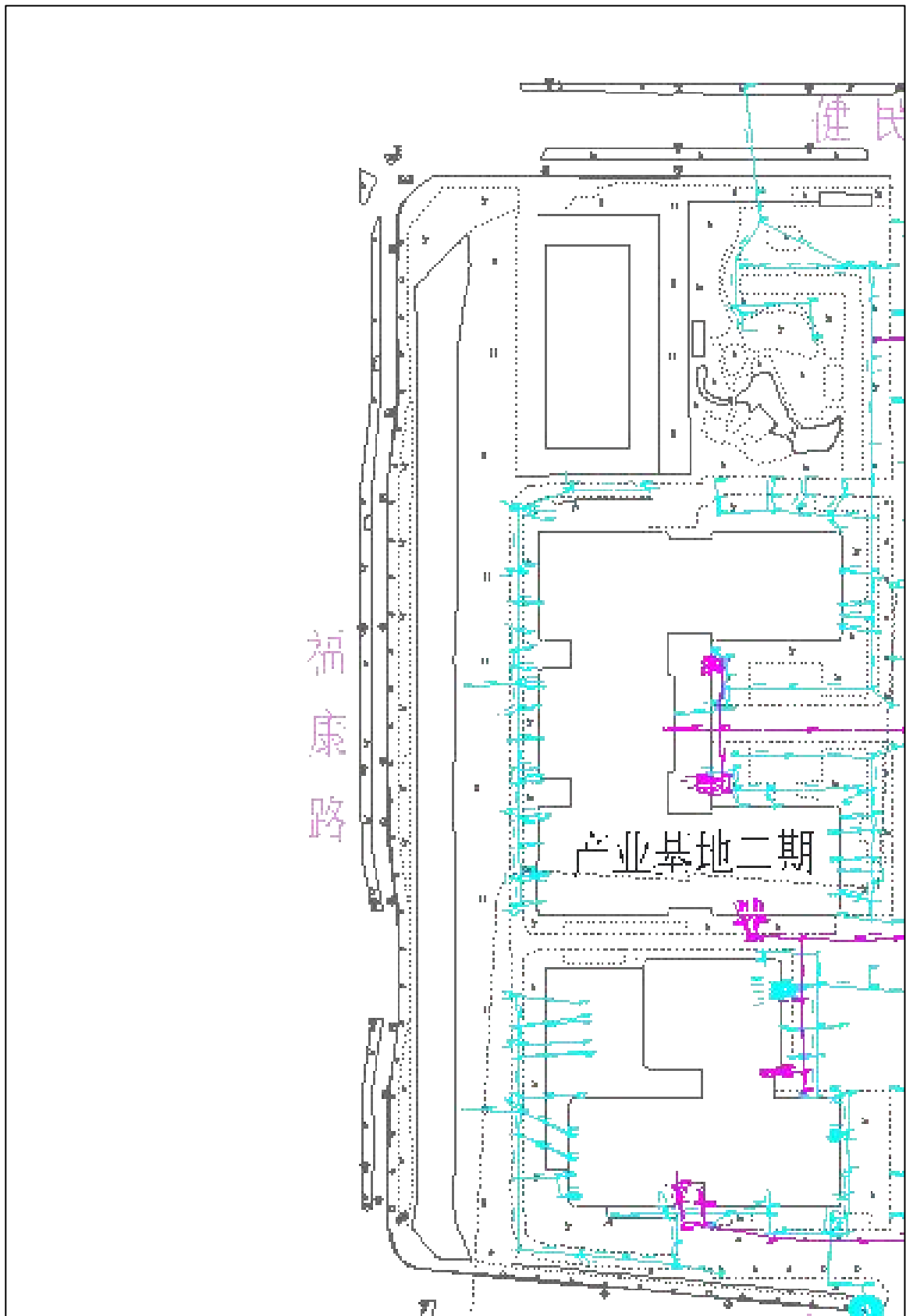
附图 4 建设项目雨污水管网及雨污水排口图
